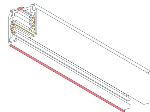
Ansicht auf Stromschienenrückseite Rote Linie zeigt die erhöhte Kante
