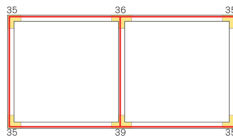
Ansicht auf Stromschienenrückseite Rote Linie zeigt die erhöhte Kante
