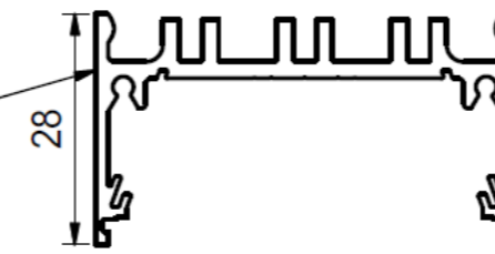
KD PROFIL 1-FACH
