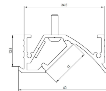
KF PROFIL
