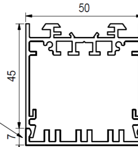
KD LEUCHTENPROFIL
